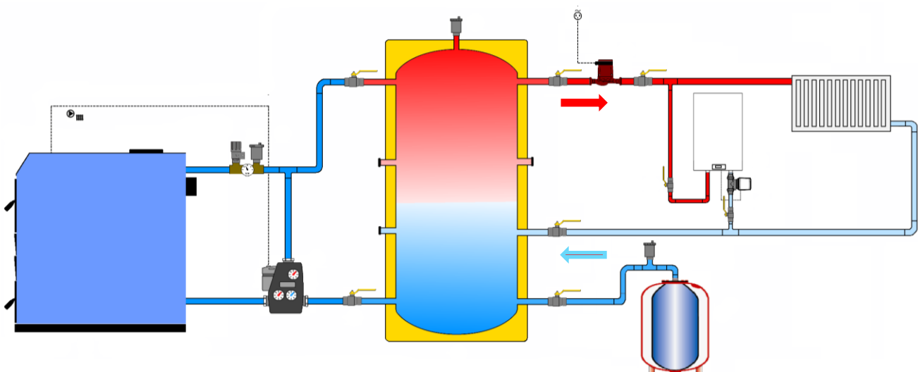
Systemfase. Lagertank afgiver varme bund til top
