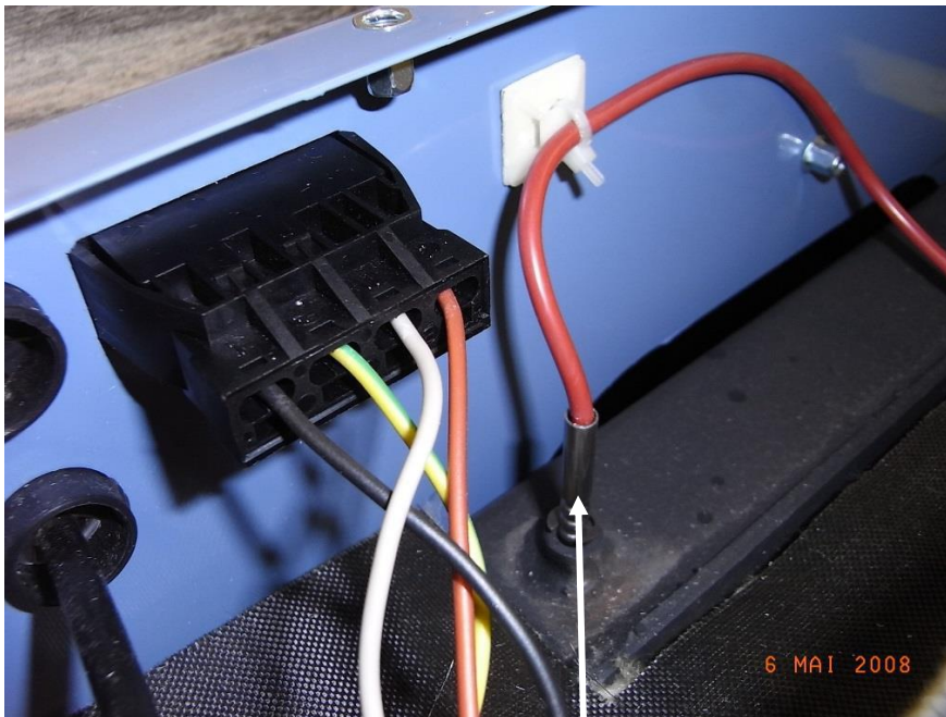
Røggastemperaturføler
